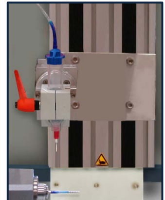
Druckbasiertes Farbdosiersystem
