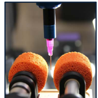
Reinigungseinrichtung für Dosiernadel
